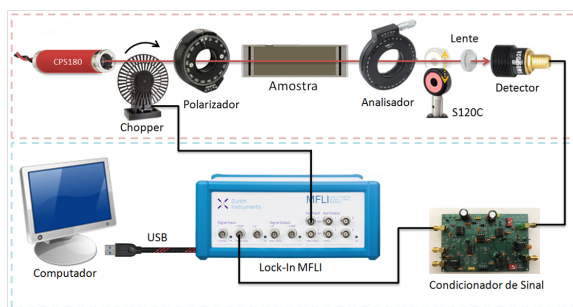
Figura 3: Aparato experimental para medidas de atividade ótica utilizando o Lock-in MFLI
