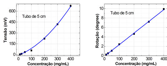
Figura 10: Resultados obtidos utilizando um caminho óptico de 5 cm. Em (a) temos a resposta da tensão para diferentes concentrações. Em (b) temos a rotação óptica referente a cada amostra.
