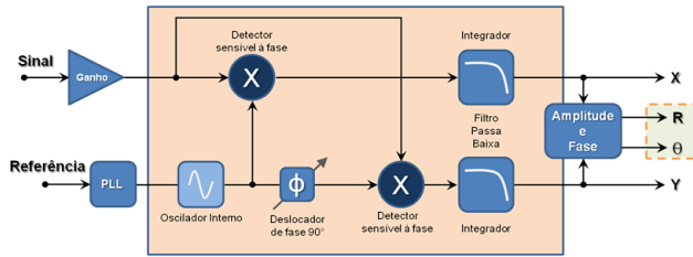
Figura 6: Diagrama em blocos do funcionamento de um amplificador Lock-in.
