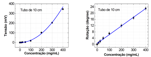
Figura 9: Em (a) temos a tensão em função da concentração da amostra e em (b) o ângulo de rotação ótica em função da concentração amostra.
