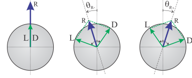
Figura 2: Representação da luz ao atravessar uma substância opticamente ativa. A onda resultante linear sofre rotação do seu plano de polarização para a esquerda ou para a direita dependendo dos índices de refração relativos às componentes circulares.
