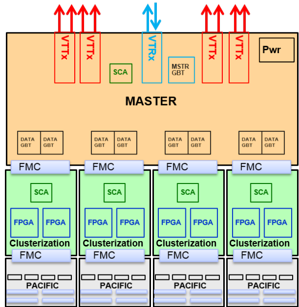
Figura 3: Diagrama ilustrando módulos que compõem a eletrônica de front-end .
