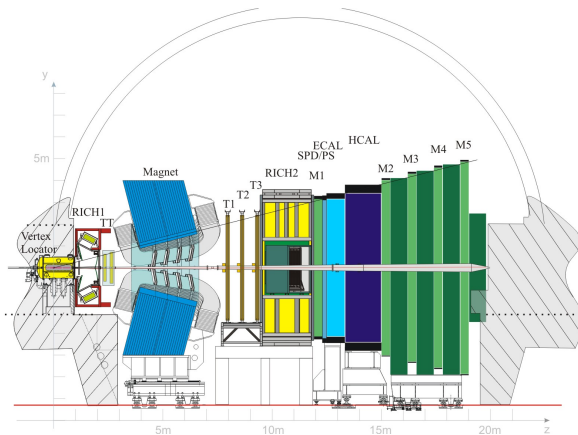
Figura 1: Vista lateral do detector LHCb.
