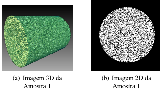
Figura 11: Imagens 3D (à esquerda) e imagem do conjunto de imagens 2D (à direita) da Amostra 1
