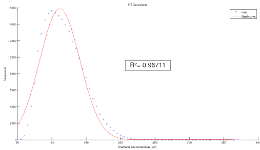
Figura 15: Fit Gaussiano - Método K-means da Amostra (1). É possível observar o coeficiente de correlação entre as curvas muito próximo de 1, indicando qualidade no ajuste entre os dados.
