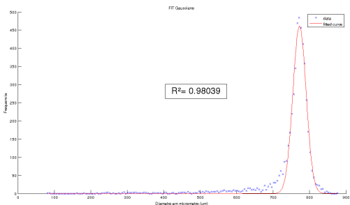
Figura 18: Fit Gaussiano - Método Entropia Local da Amostra (2). É possível observar o coeficiente de correlação entre as curvas muito próximo de 1, indicando qualidade no ajuste entre os dados.
