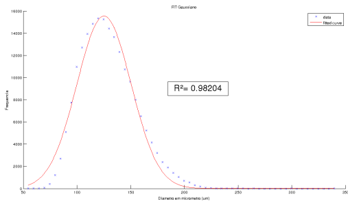
Figura 14: Fit Gaussiano - Método Otsu da Amostra (1). É possível observar o coeficiente de correlação entre as curvas muito próximo de 1, indicando qualidade no ajuste entre os dados.
