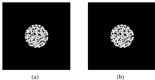
Figura 20: Imagens de microesferas de 780 micrômetros segmentadas pela técnica Entropia Local (esquerda) e K-means (direita).
