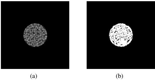
Figura 19: Exemplo de imagem original corrigida por contraste a após filtro mediano (esquerda) e segmentação de imagem da amostra de 780 micrômetros pelo método Otsu (direita). É possível notar que a segmentação não permitiu visualizar contornos de muitas microesferas.
