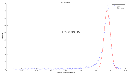
Figura 17: Fit Gaussiano - Método K-means da Amostra (2). É possível observar o coeficiente de correlação entre as curvas muito próximo de 1, indicando qualidade no ajuste entre os dados.
