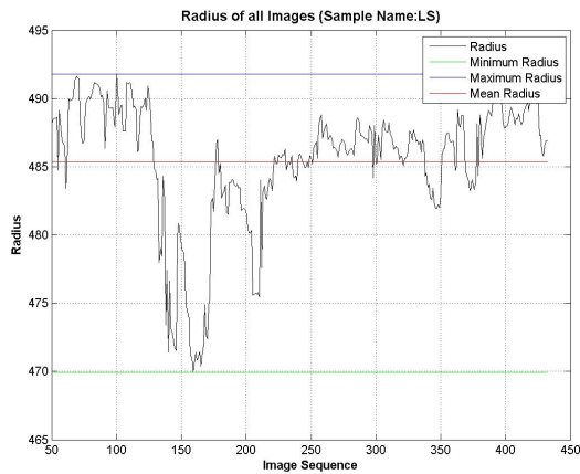
Figura 3: Gráfico que relaciona um conjunto de imagens do reservatório LS (i.e. Lagoa Salgada) com o raio original de cada uma delas. Demonstra o impacto na determinação de cada tipo de raio, destacados nas cores azul, vermelha e verde, definidos para a ROI.
