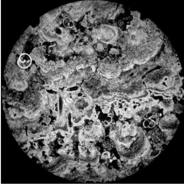
Figura 1: Imagem Micro-CT, fornecida pelo CENPES, de amostra retirada do reservatório de Lagoa Salgada localizado no litoral norte do Estado do Rio de Janeiro.
