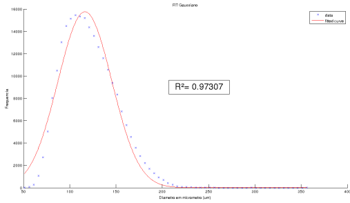
Figura 16: Fit Gaussiano - Método Entropia Local da Amostra (1). É possível observar o coeficiente de correlação entre as curvas muito próximo de 1, indicando qualidade no ajuste entre os dados.
