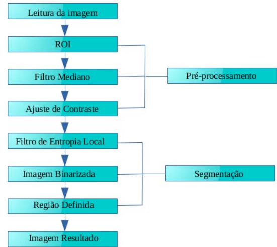
Figura 2: Diagrama das etapas de processamento do algoritmo. A primeira etapa prepara a imagem. Esse pré-processamento delimita a ROI. Utiliza o filtro mediano e o ajuste de contraste para definir melhor os contornos auxiliando o processo de segmentação, que tem como principal o filtro de Entropia Local. A região binarizada resultante é definida por máscara na imagem original, separando a fase de interesse e descartando o restante da imagem.
