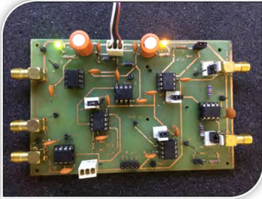
Figura 16: Placa de um circuito condicionador de sinal desenvolvida no LEPS do CBPF usando a técnica do dryfilm .
