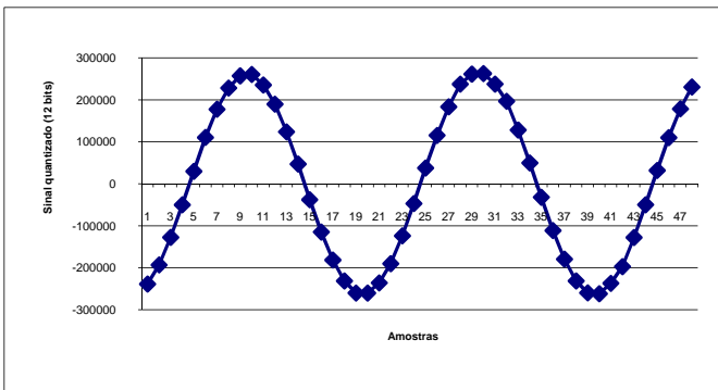
Figura 17: Produto dos sinais de entrada e referencia em quadratura.
