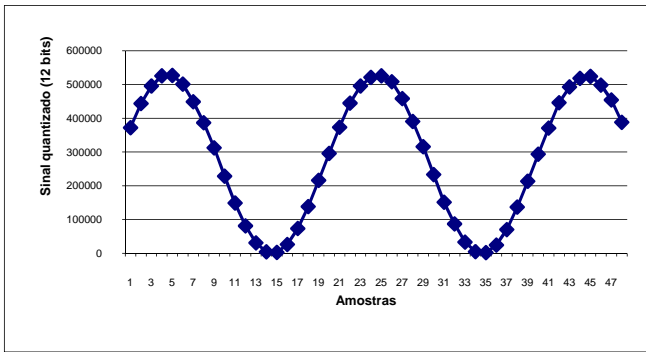
Figura 16: Produto dos sinais de entrada e referencia estando ambos em fase.
