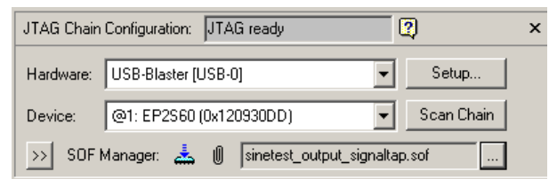
Figura 9: Carregando o arquivo .sof dentro do Quartus II.
