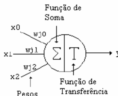
Figura 3.1 Neurônio Artificial
