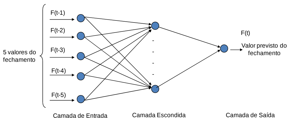
Figura 4.3 Arquitetura proposta.
