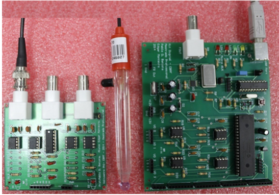
Figura 4: Placa de controle e aquisição de dados e placa de caracterização elétrica do EGFET
