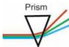
Fig. 2 – Separação de um feixe de luz em cores
