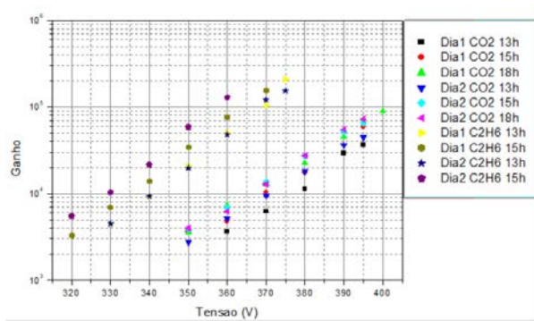
Figure 6: Reprodutibilidade da Curva de ganho para diferentes combinações gasosas.
