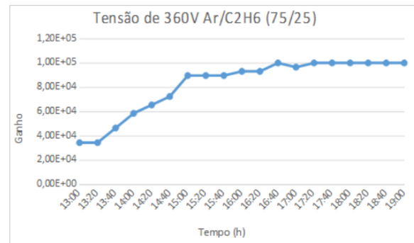
Figure 8: Variação do ganho usando um pré-amplificador de carga, durante seis horas, para a mistura gasosa \text{Ar}/\text{C}_2\text{H}_6(75/25) .
