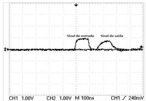
Figure 13: Sinais na entrada e na saída da linha de retardo \tau . O atraso total da linha é de aproximadamente 160 ns.
