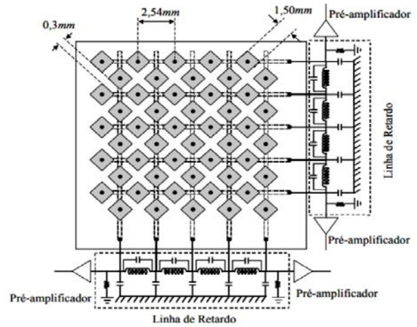
Figure 3: Anodo X&Y com linha de retardo.
