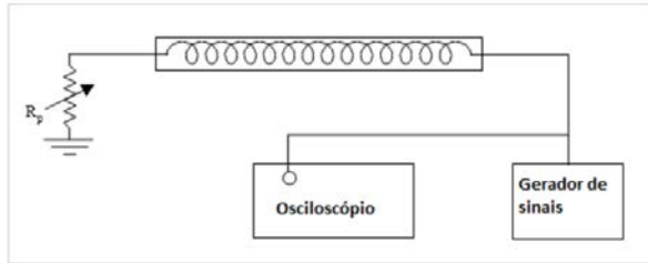
Figure 9: Esquema usado para determinar a impedância característica da linha de retardo.
