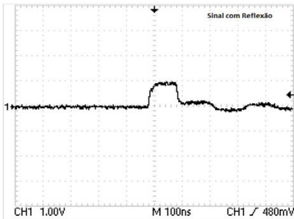
Figure 10: Pulso enviado e pulso refletido observados no osciloscópio.
