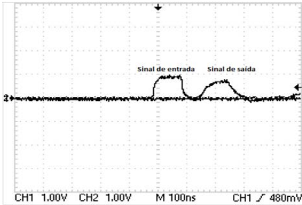
Figure 14: Sinais na entrada e na saída da linha de retardo X. O atraso total da linha é de aproximadamente 160 ns.
