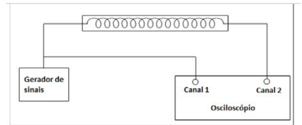
Figure 12: Esquema usado para determinar o atraso total da linha de retardo.
