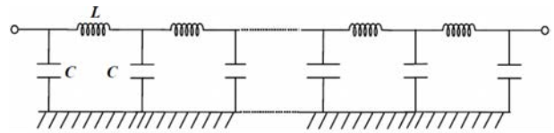
Figure 4: Circuito de uma linha de retardo discreta composta por filtros LC.
