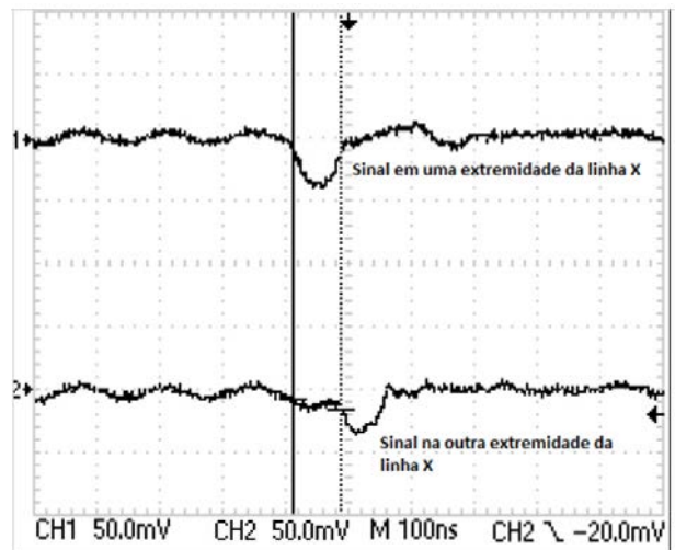
Figure 16: Sinais observados na saída dos pré-amplificadores de tensão.
