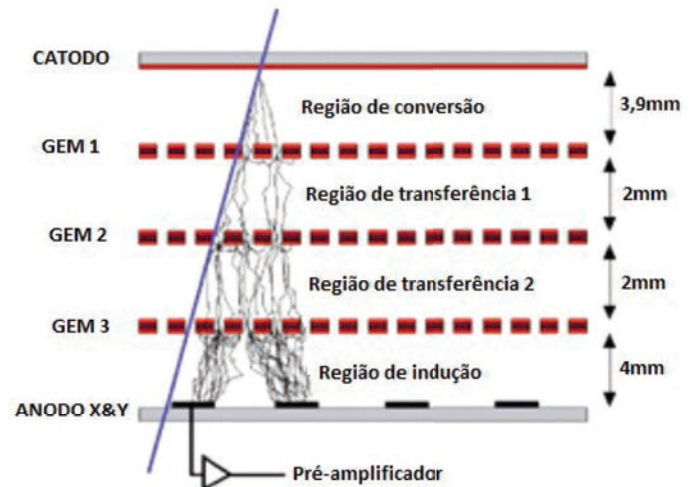
Figure 1: Imagem do dispositivo triplo-GEM.
