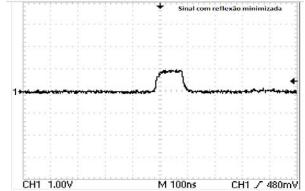
Figure 11: Sinal com reflexão minimizada observado no osciloscópio.
