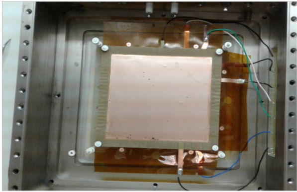
Figure 2: Montagem do dispositivo triplo-GEM.
