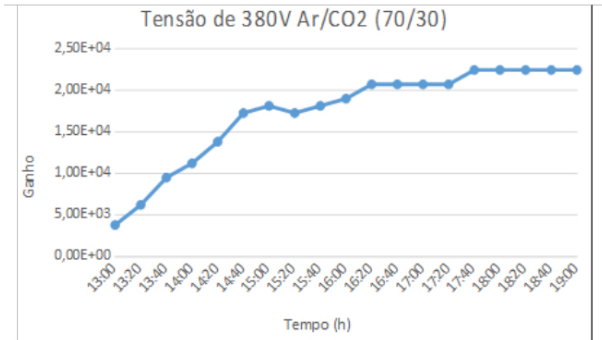
Figure 7: Variação do ganho usando um pré-amplificador de carga, durante seis horas, para a mistura gasosa \text{Ar}/\text{CO}_2(70/30) .
