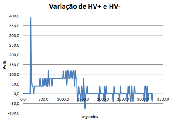
Figura 20 - Gráfico da variação de HV até estabilização em 10KV.
