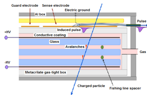
Figura 1a – Corte transversal de um detector RPC.
