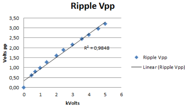
Figura 21 – Ripple de tensão de saída.
