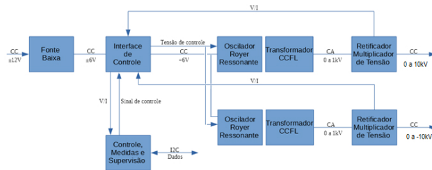
Figura 2 – Diagrama em blocos da fonte HVPS-CBPF.
