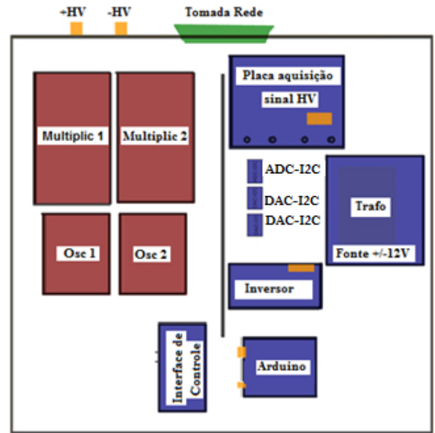
Figura 4a – Protótipo montado em rack de 40 cm × 40 cm.
