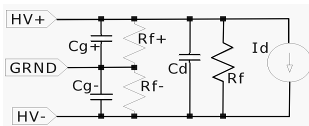
Figura 1b – Circuito eletrônico equivalente.
