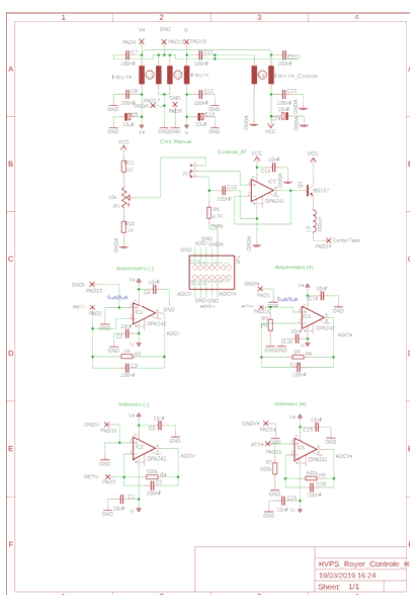
Figura 8 – Placa de leitura e controle original.
