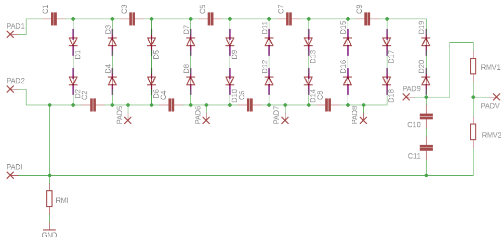
Figura 6 – Esquema elétrico do Retificador Multiplicador de Voltagem Negativo – CDVM.
