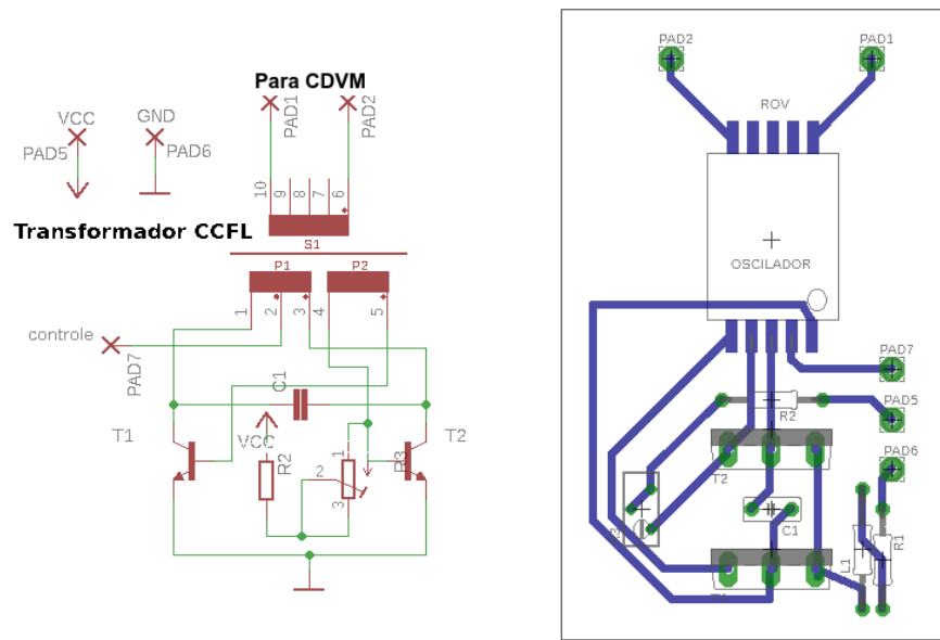
Figura 5 – Placa de circuito impresso do oscilador Royer.
