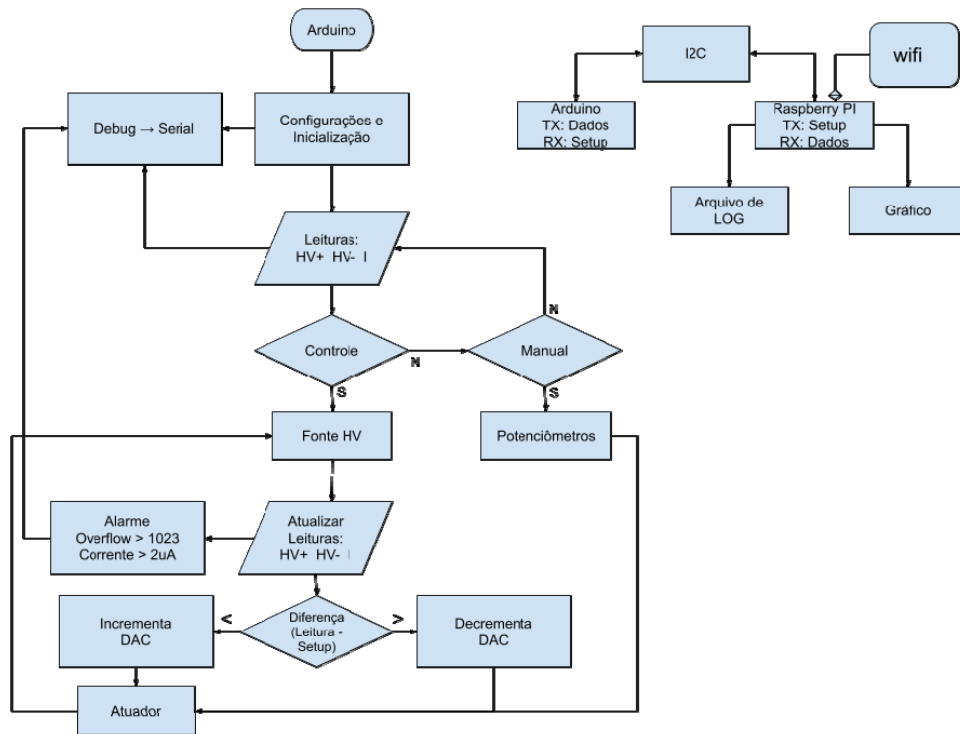
Figura 18 - Diagrama do sistema de controle Raspberry/Arduíno.
