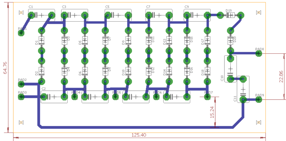
Figura 7 – Layout do Retificador Multiplicador de Voltagem Negativo – CDVM.
