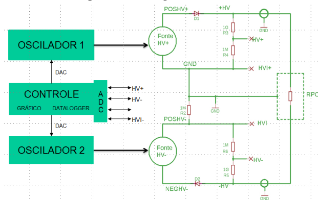
Figura 3 – Interface para ADC do circuito de amostragem das tensões e correntes.
