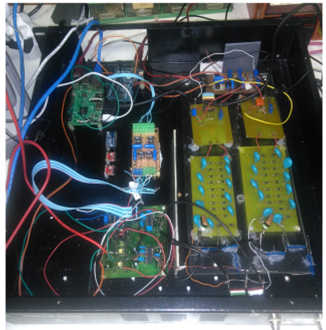
Figura 4b – Foto do protótipo em bancada.
