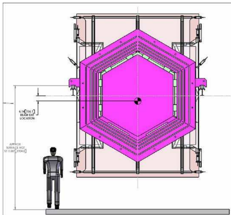
Figura 3.7: Vista do detector do MINER \nu A ilustrando forma e tamanho. A estrutura alta, parcialmente encoberta pelo detector, é a parede de veto
