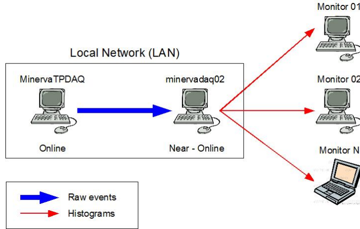
Figura 5.1: Esquema geral do software de aquisição de dados do MINERνA.
