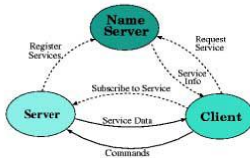
Figura C.2: Diagrama de fluxo de dados do DIM
