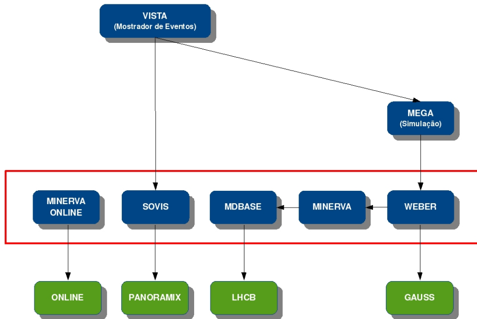
Figura 4.3: Detalhes da dependência do software do MINER \nu A v3r1 com o software do LHCb em maio 2009. Azul: software específico do MINER \nu A. Verde: software do LHCb.
