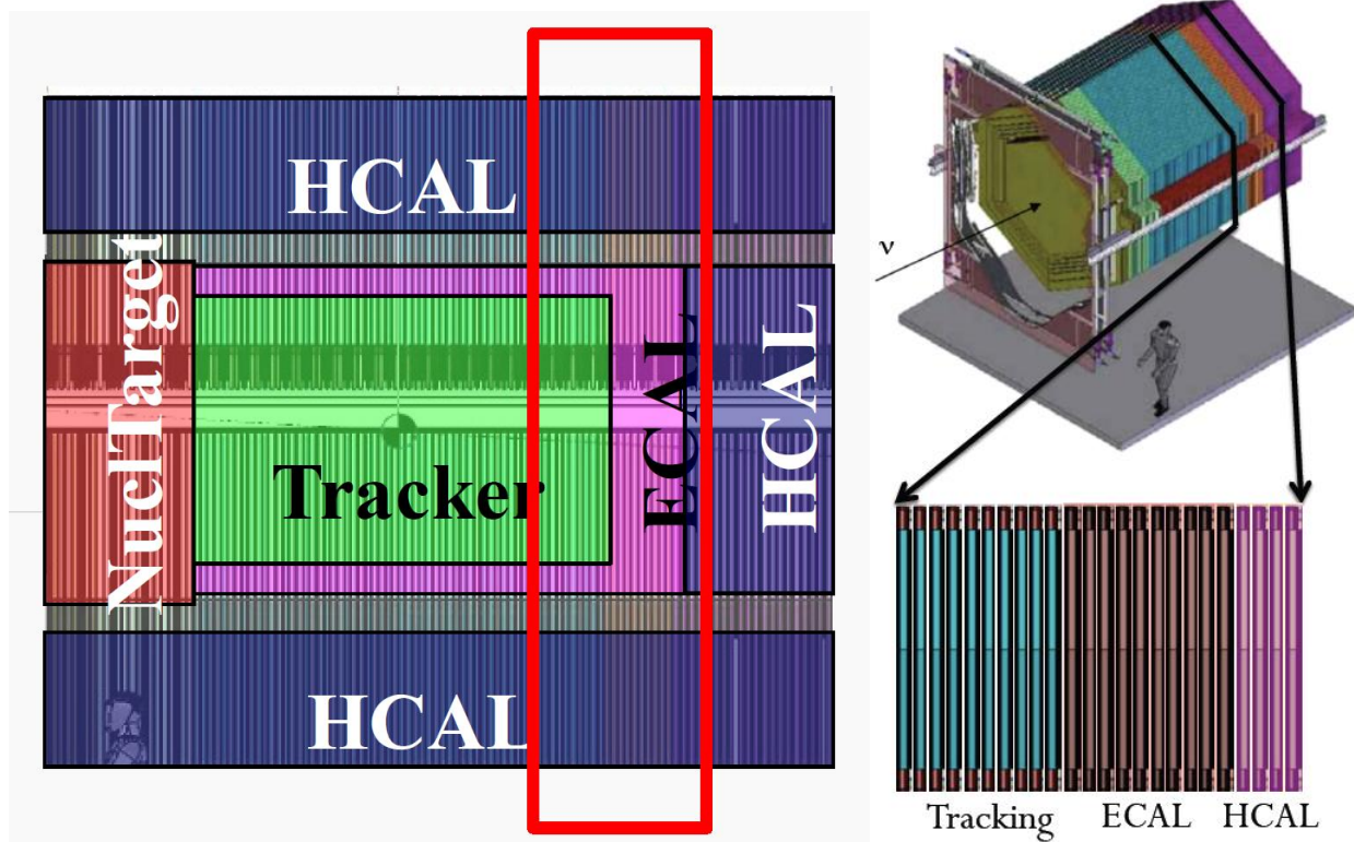
Figura 3.19: Esquema do detector de do MINER \nu A mostrando a parte que corresponde ao protótipo de rastreamento
