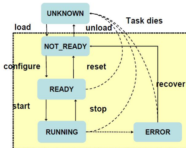
Figura C.3: Diagrama de estados dos processos rodando como programas GAUDI online .
