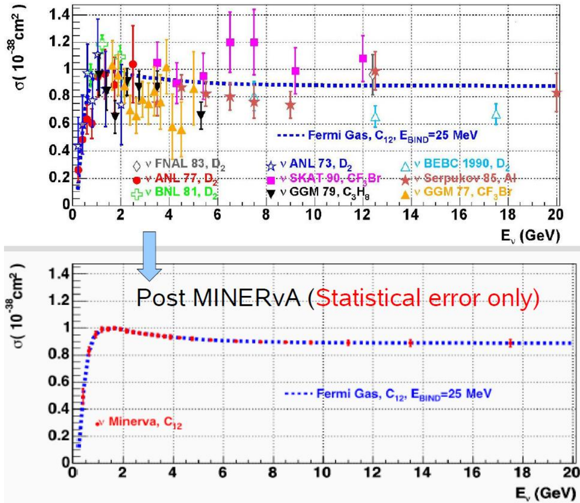
Figura 3.21: superior: Previsão dos resultados de medida da seção de choque quase-elástica esperada pelo MINER \nu A (apenas erros estatísticos). inferior: medidas atuais da seção de choque quase-elástica. A linha pontilhada em azul emprega um modelo de gás de Fermi.
