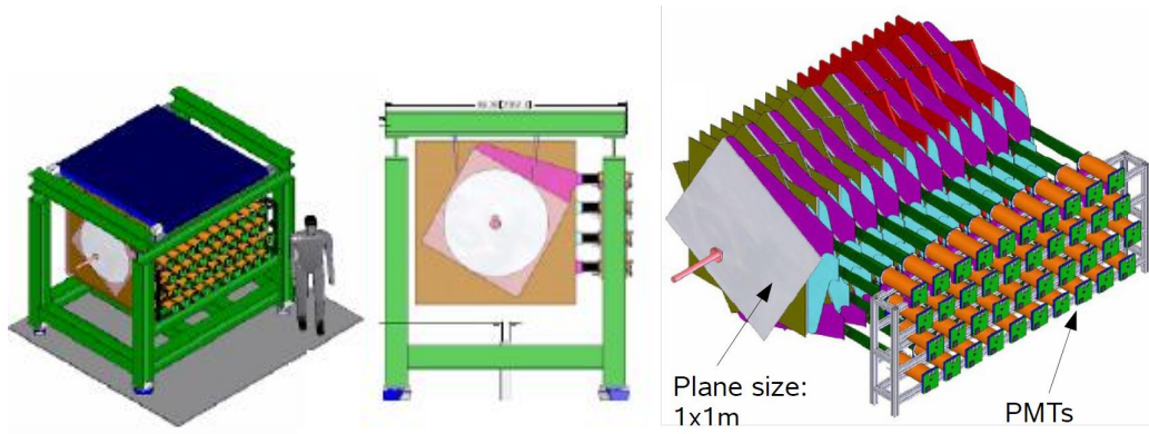
Figura 3.18: O detector de provas do MINER \nu A .
