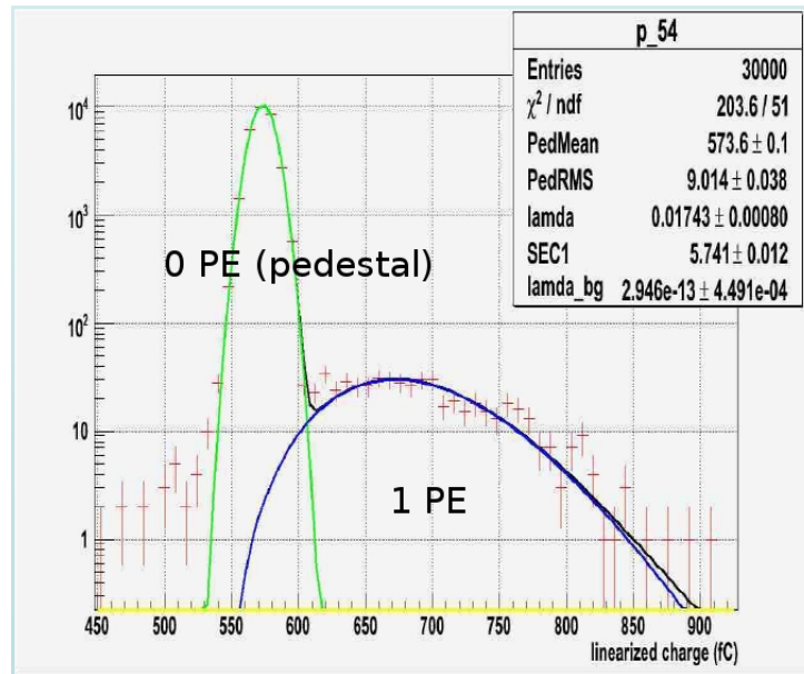
Figura 6.13: Resultados obtidos usando a distribuição OnePE. Cortesia de Brandon Eberly, University of Pittsburgh
