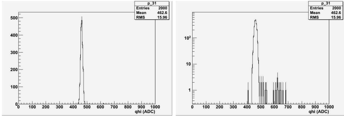
Figura 6.9: Uma distribuição de pedestal comum obtida a partir de um só canal das PMTs. A amplitude do sinal (carga coletada) é apresentada em contagens de ADC. O lado direito apresenta a mesma distribuição em escala logarítmica.
