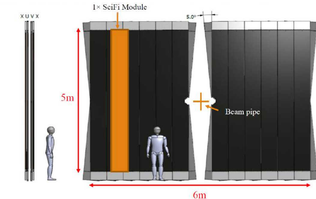
Figura 5.2: Modelo 3D do arranjo dos módulos do detector SciFi.
