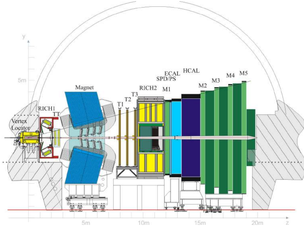
Figura 3.1: Vista lateral do detector do experimento LHCb.
