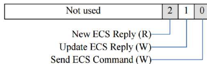
Figura 9.8: Ilustração do registrador de controle utilizado pelo bloco SOL40_SCA.
