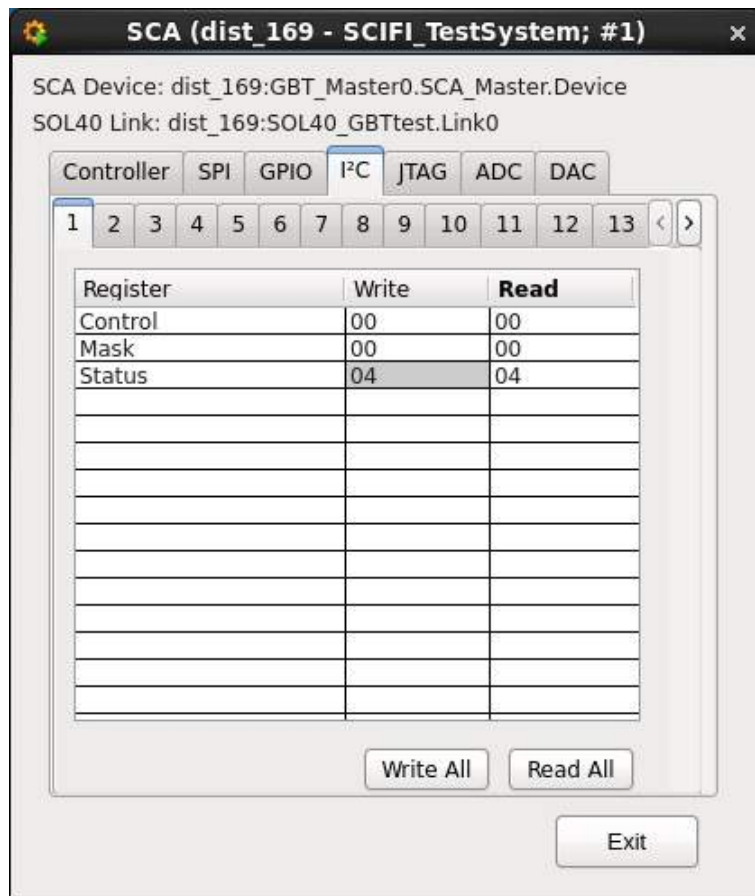
Figura 9.16: Painel desenvolvido para leitura e escrita nos registradores do GBT SCA.
