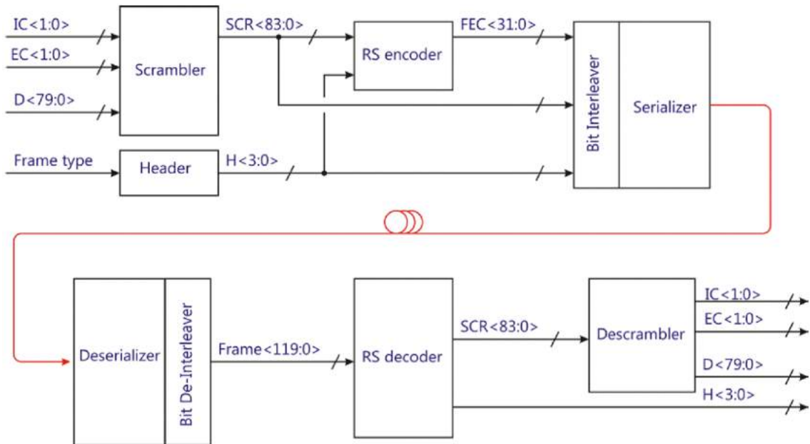
Figura 4.4: Diagrama de blocos do codificador e decodificador do GBT-FPGA.
