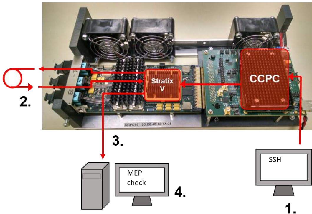
Figura 8.9: Teste de envio e aquisição de dados em loopback.
