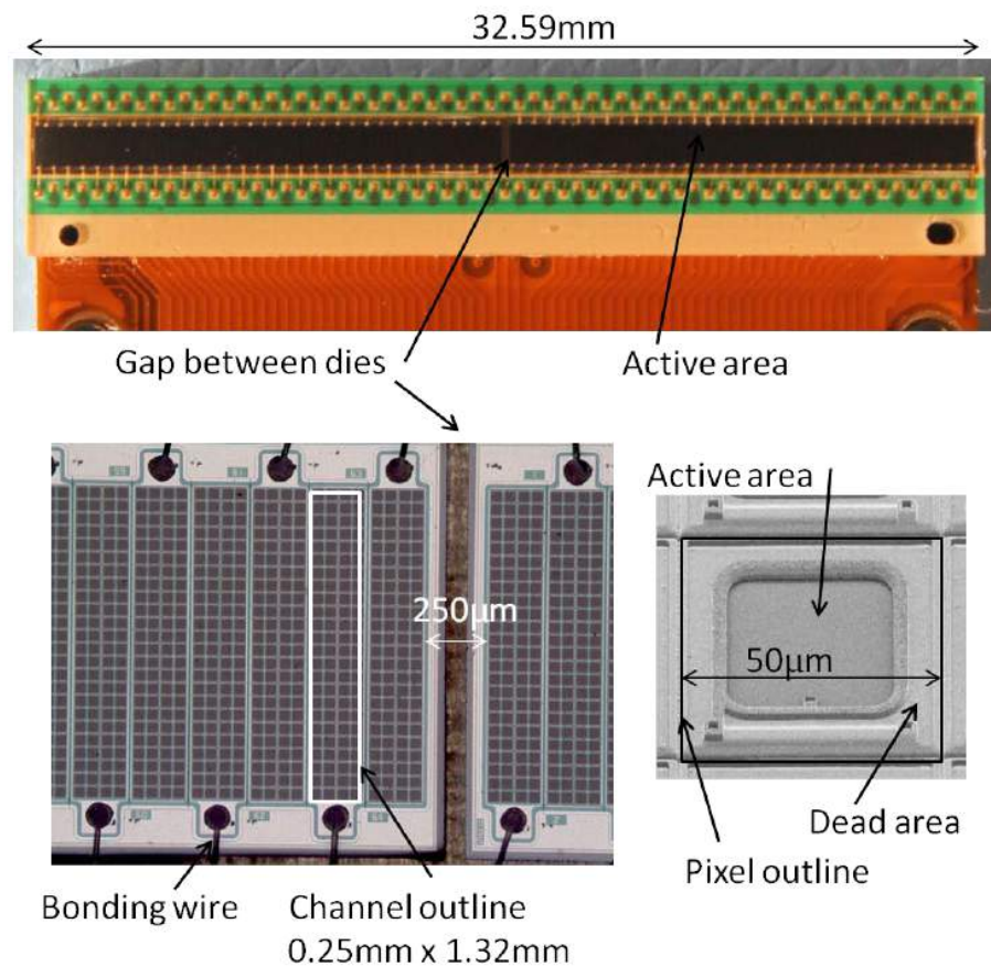
Figura 5.7: Topo: encapsulamento do sensor com 2 pastilhas de silício. Inferior esquerda: ampliação da parte central do sensor, onde se pode ver os canais individuais e o intervalo espacial entre eles. Inferior direita: ampliação de um único pixel.
