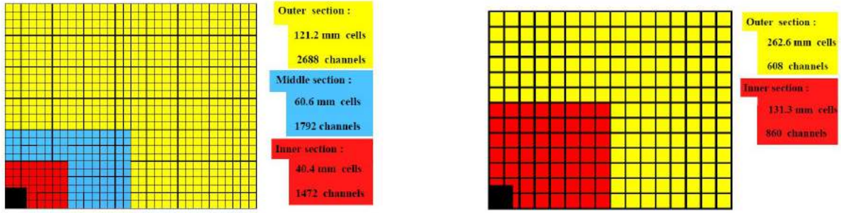
Figura 3.7: Ilustração da granularidade nos SPD, PS e ECAL (esquerda) e no HCAL (direita).
