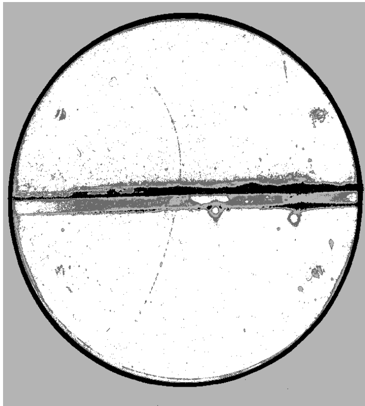
Figura 1: Fotografia do traço de ionização deixado por um pósitron em uma câmera de nuvem no experimento de Anderson ao atravessar uma placa de chumbo de 6 mm.
