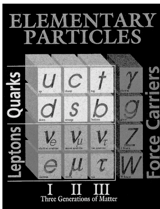
Figura 3: Tabela das Partículas Elementares de hoje segundo material divulgado pelo Fermilab, por ocasião da descoberta do quark top.
