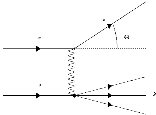
Figura 2: Esquema para o Espalhamento Profundamente Inelástico, do elétron ( e ) pelo próton ( p ), visto no laboratório onde o próton está em repouso.
