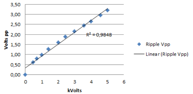
Figura 21 – Ripple de tensão de saída.
