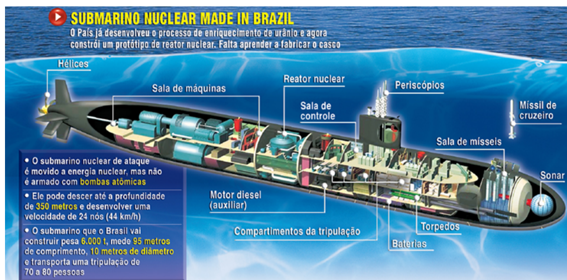
Fig. 11. PROSUB-Projeto do Submarino a propulsão nuclear da Marinha do Brasil.
