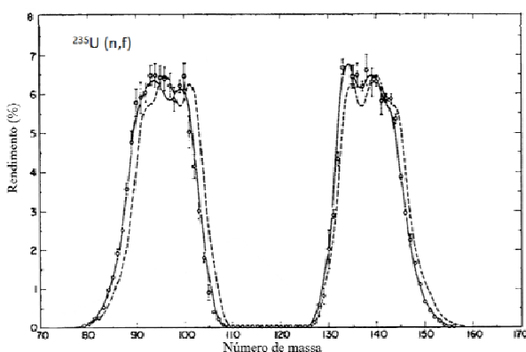
Fig. 7. Distribuição de massa de fragmentos primários — i. e. , antes da emissão imediata de nêutrons— (curva tracejada) e de produtos de fissão— i. e. , após a emissão de nêutrons—(curva contínua) na fissão de ^{235}\text{U} induzida por nêutrons (adaptado de [42]).
