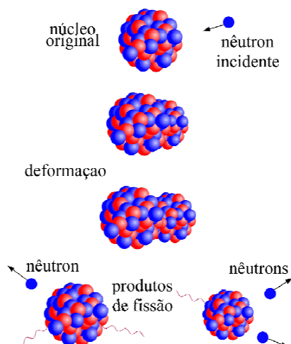
Fig. 1. Bipartição de um núcleo pesado (urânio ou tório) por incidência de um nêutron.
