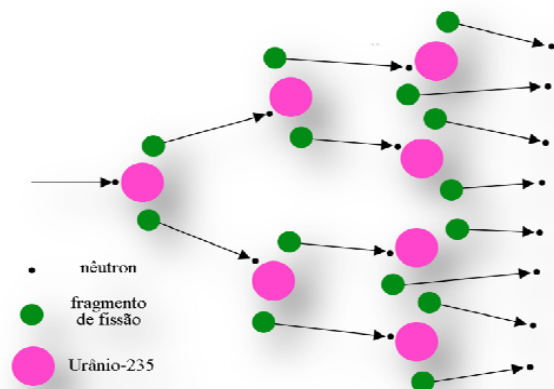
Fig. 2. Esquema das reações de fissão nuclear em cadeia.
