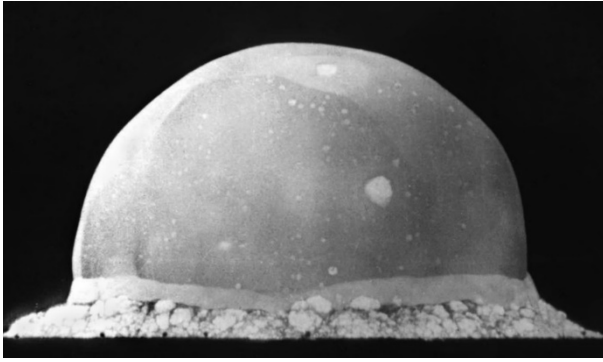
Fig. 5. Imagem da detonação da 1ª bomba atômica (o Teste Trinity) acionada em 16 de julho de 1945 em Alamogordo (Novo México, EUA); construída à base de ^{239}\text{Pu} , liberou 23 GWh.
