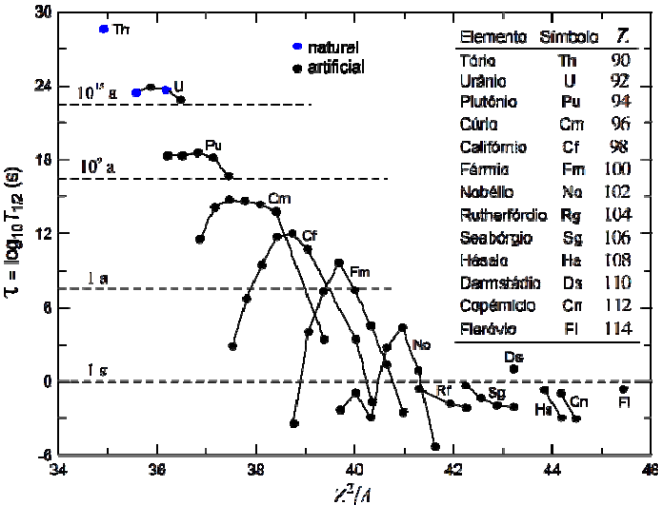
Fig. 3. Meia-vida por fissão espontânea de núcleos pesados da natureza (urânio e tório) e artificiais (dados extraídos de [36]).
