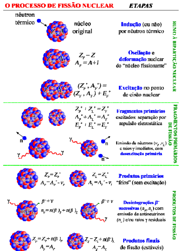
Fig. 6. Etapas do processo de bipartição nuclear (extraído de [41]).
