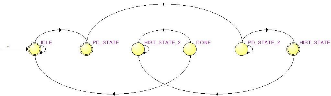
Figure 5: Máquina de Estados do bloco MCA_comp
