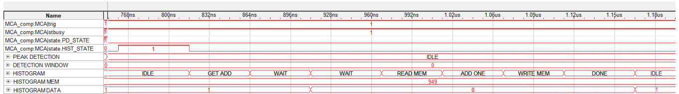
Figure 14: Comportamento verificado do bloco de gerenciamento da memória
