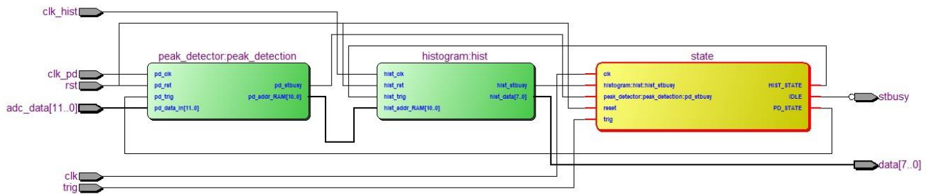
Figure 4: Diagrama em blocos do componente “MCA_comp”
