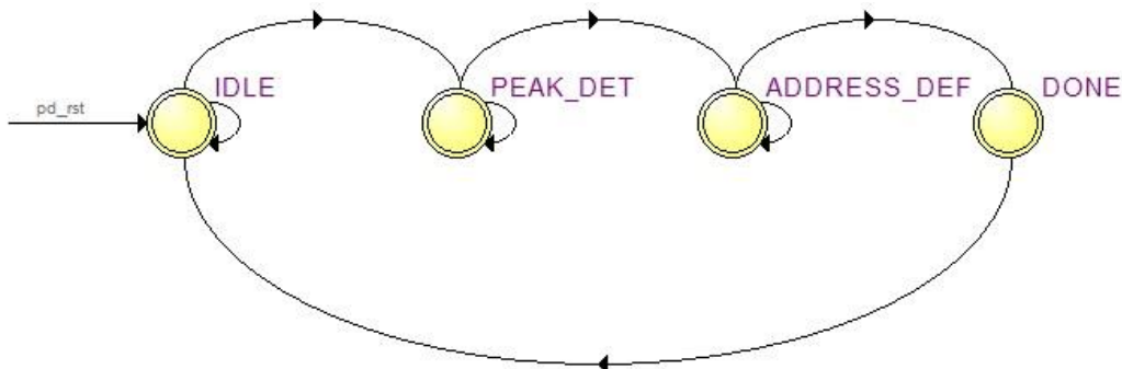
Figure 6: Máquina de Estados do bloco “peak_detector”
