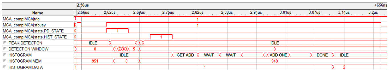
Figure 15: Comportamento do MCA em um Segundo evento de mesma energia
