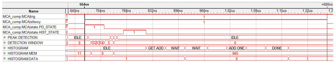
Figure 12: Comportamento geral verificado do MCA
