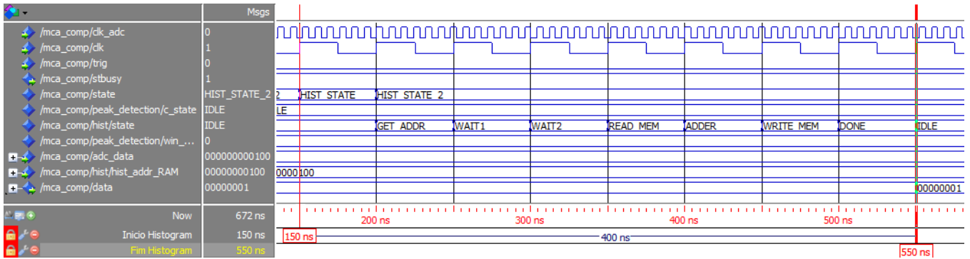
Figure 9: Simulação do código programado - gerenciamento de memória Fonte: (LSD, CBPF)
