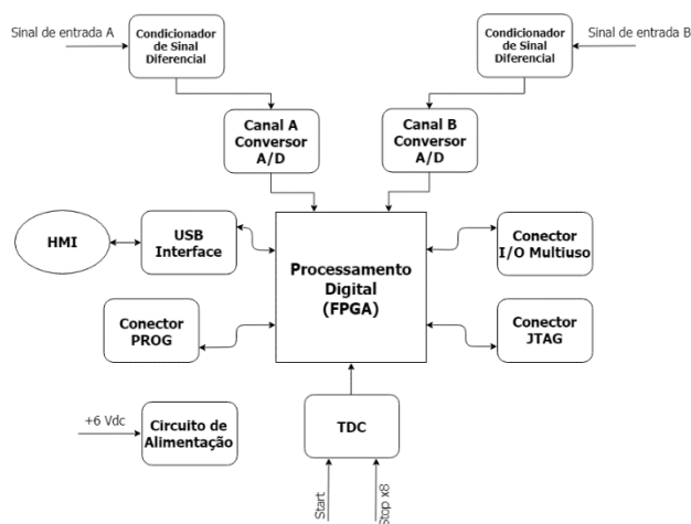
Figure 2: Diagrama em blocos do SPRO Fonte: (LSD, CBPF)
