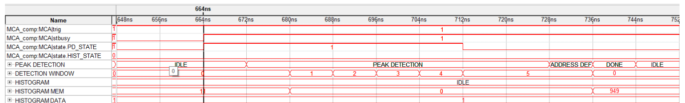
Figure 13: Comportamento verificado do bloco de detecção de pico
