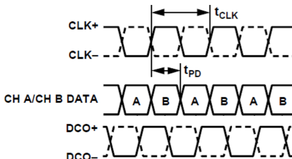
Figure 3: Diagrama de onda ADC9627-125 Fonte: ( http://www.analog.com )
