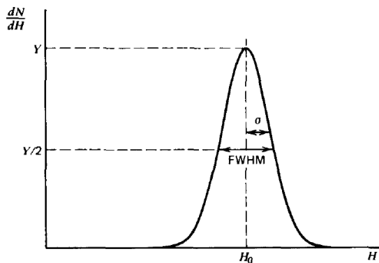
Figure 1: Definição da resolução de um detector.
