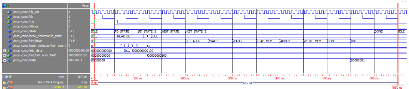
Figure 10: Simulação do código programado do MCA Fonte: (LSD, CBPF)
