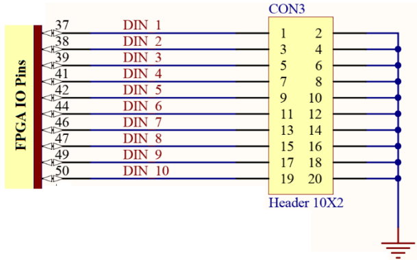
Figure 11: Conector de entradas e saídas digitais do módulo SPRO (CON3)
