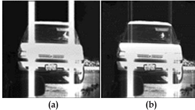
Figure 16: Efeito de blooming em duas câmeras. (a) câmera normal; (b) câmera CID.
