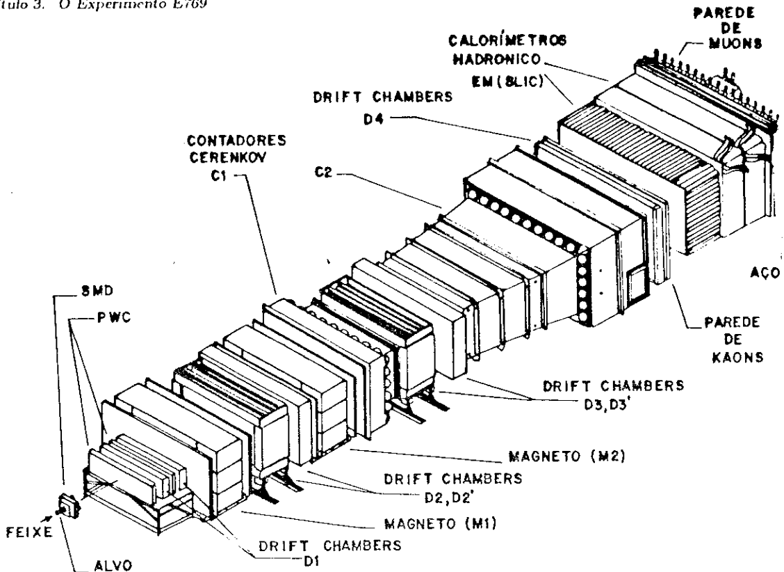
Figura 3.8: Vista em Escala do Espectrômetro da E769
