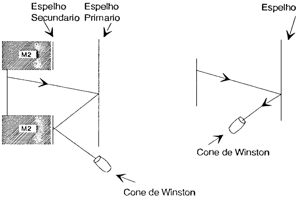
Figura 3.15: Caminho Percorrido pela Luz nos Detetores Čerenkov
