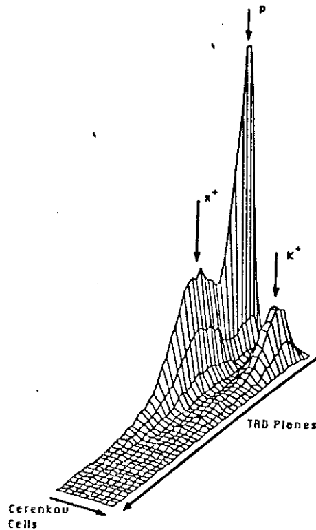
Figura 3.7: Planos Ativados do TRD versus Número de Fototubos Ativados em Coincidência no DISC
