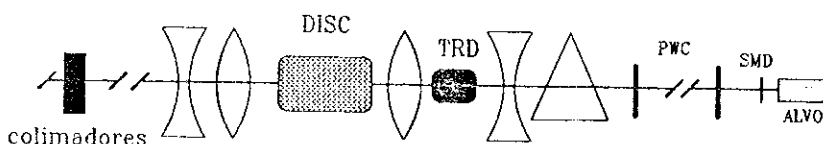
Figura 3.3: Posição do DISC e do TRD na Linha do Feixe
