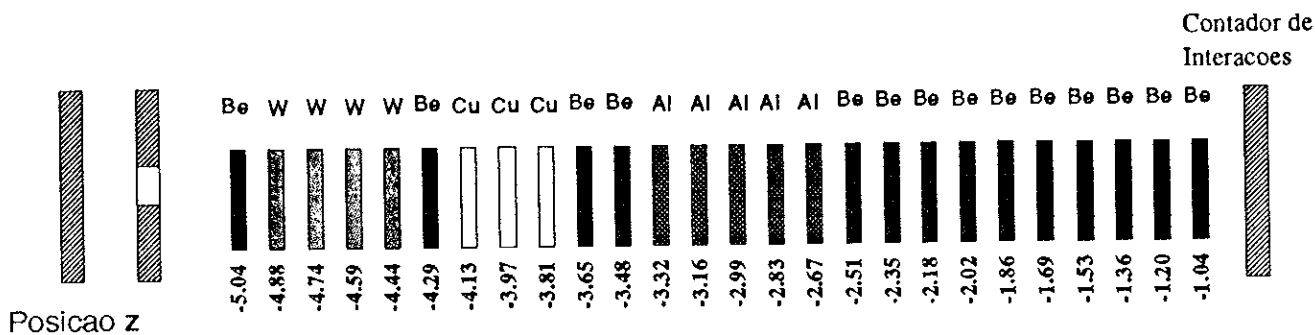
Figura 3.9: Alvo da Experiência
