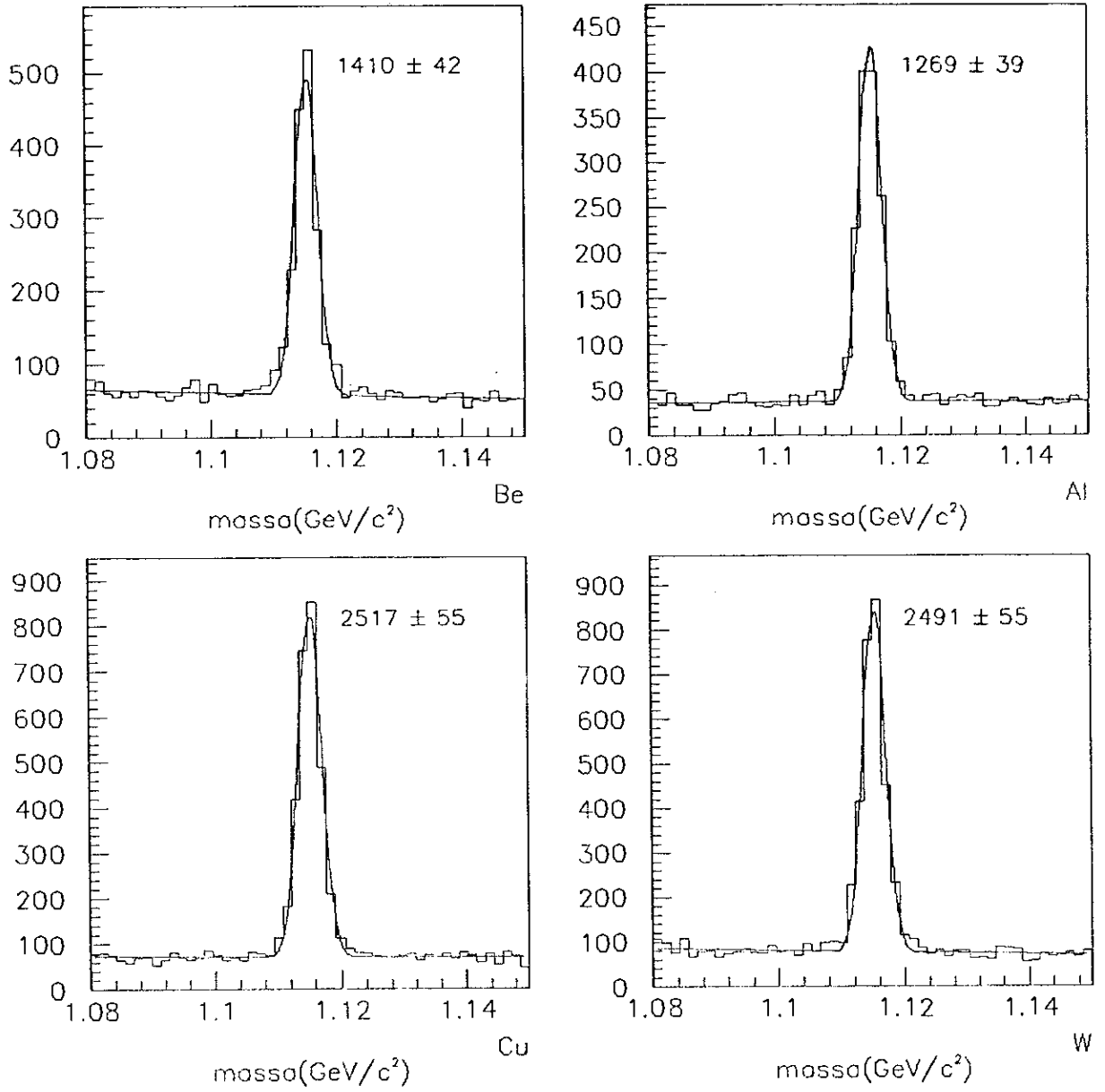
Figura 5.2: Sinais do \Lambda nos 4 Alvos da Experiência
