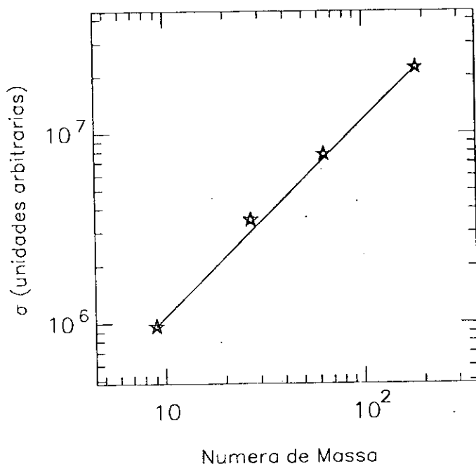
Figura 5.6: Seção de Choque versus A para o \Lambda
