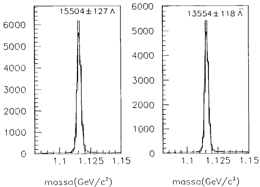
Figura 4.11: Sinais do \Lambda e \bar{\Lambda} obtidos a partir da Simulação
