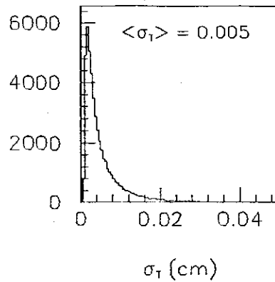
Figura 4.7: Ilustração do corte em RAT
