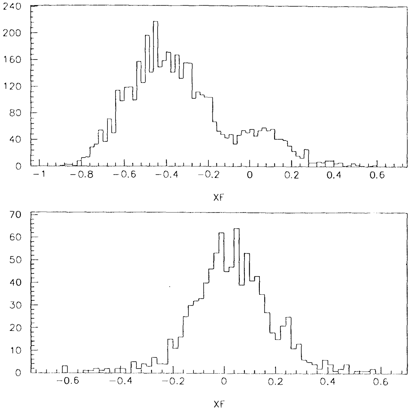
Figura 2.3: Distribuições de x_f Geradas pelo Programa de Simulação da E769 para o \Lambda (acima) e para o \bar{\Lambda} .
