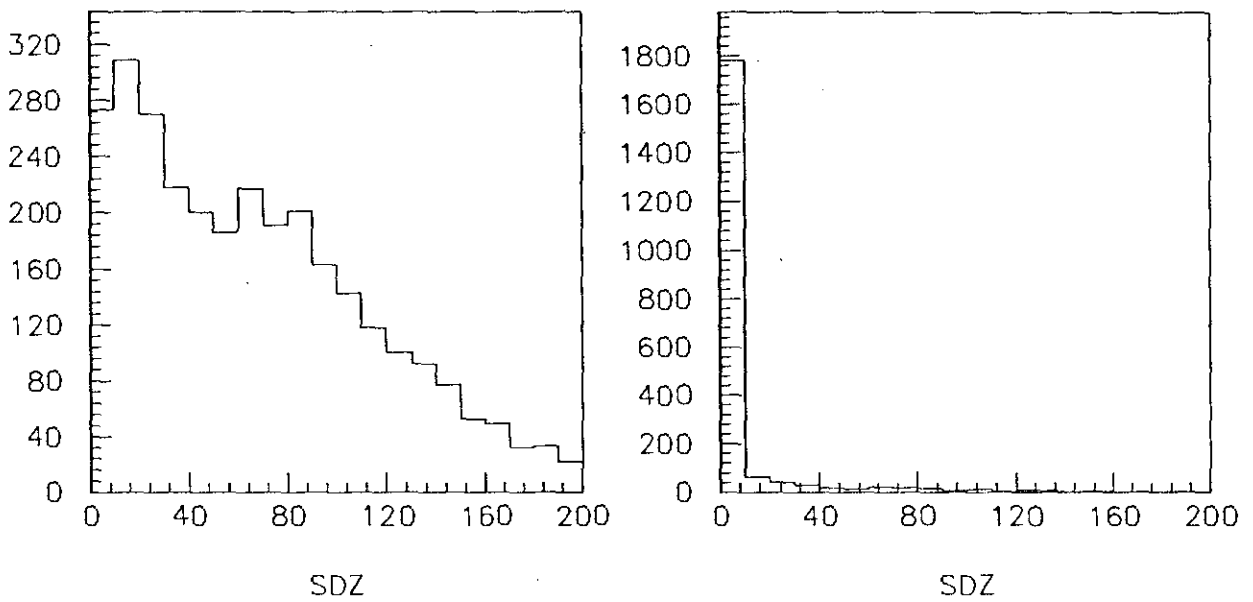
Figura 4.5: SDZ para o Sinal de MC (esquerda) e para o Background de Dados.
