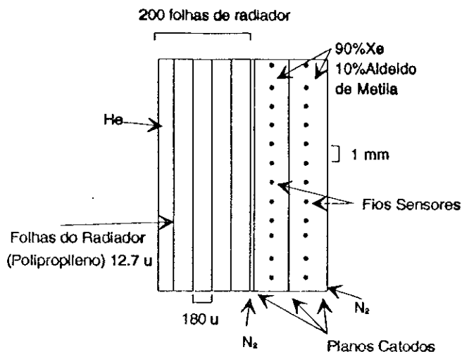
Figura 3.6: Módulo do TRD
