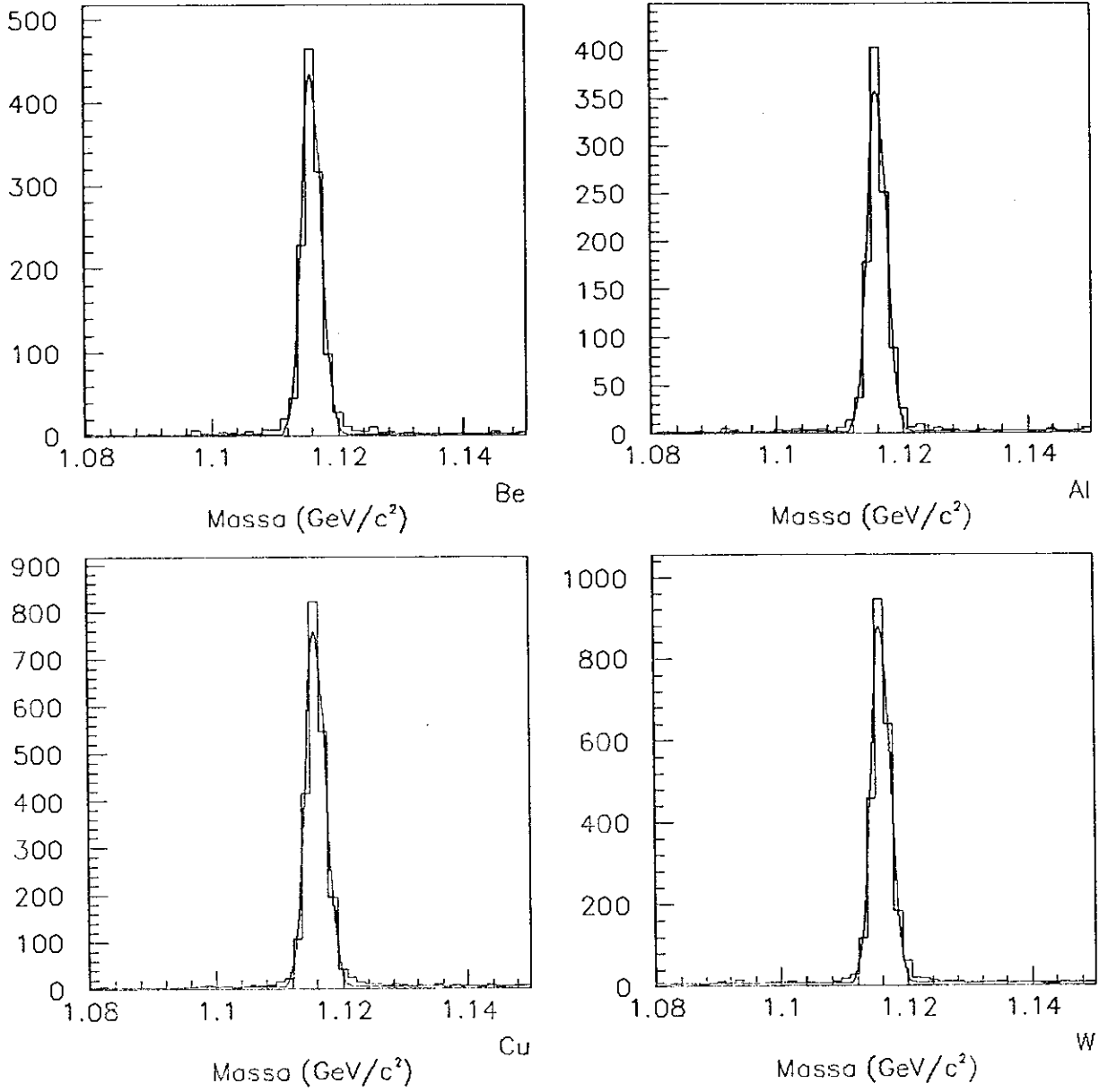
Figura 5.3: Sinais do \Lambda nos 4 Alvos da Experiência Obtidos da Simulação
