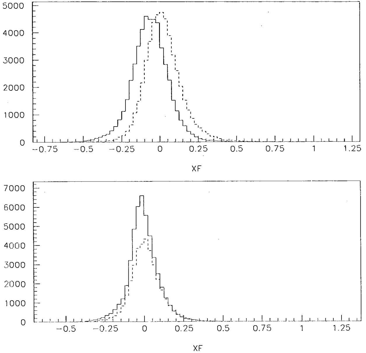
Figura 4.2: Comparação entre as Distribuições de x_f dos Dados e do MC (tracejado) para a Amostra da DC (acima) e do SMD.
