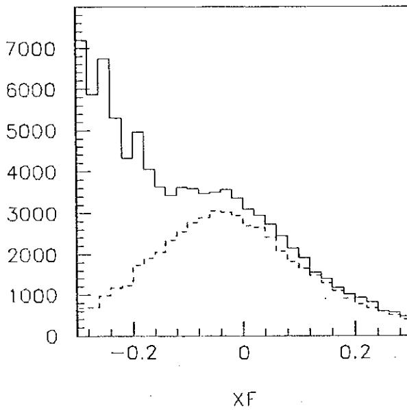
Figura 5.5: Distribuições de x_f geradas pela simulação para o \Lambda e \bar{\Lambda} (tracejado)
