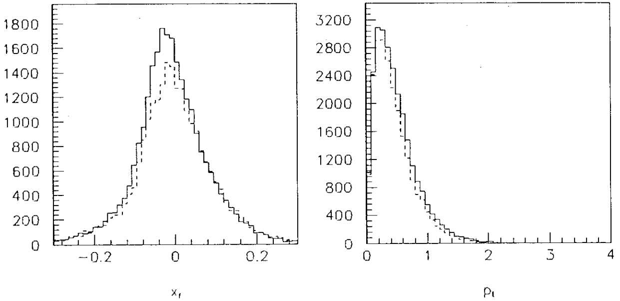
Figura 5.1: Distribuições de x_f e p_t do \Lambda e do \bar{\Lambda} (tracejado)
