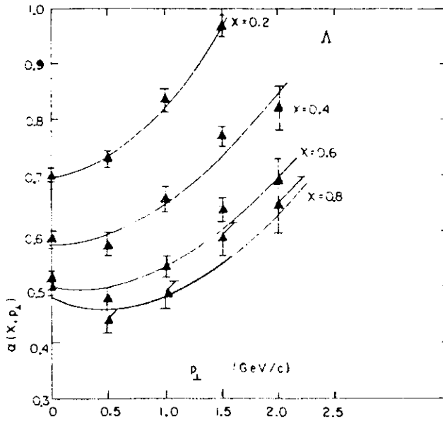
Figura 2.5: \alpha como Função de p_t para o \Lambda para Interações pA a 300 e 400 GeV/c
