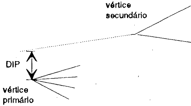
Figura 4.6: Ilustração do corte em DIP
