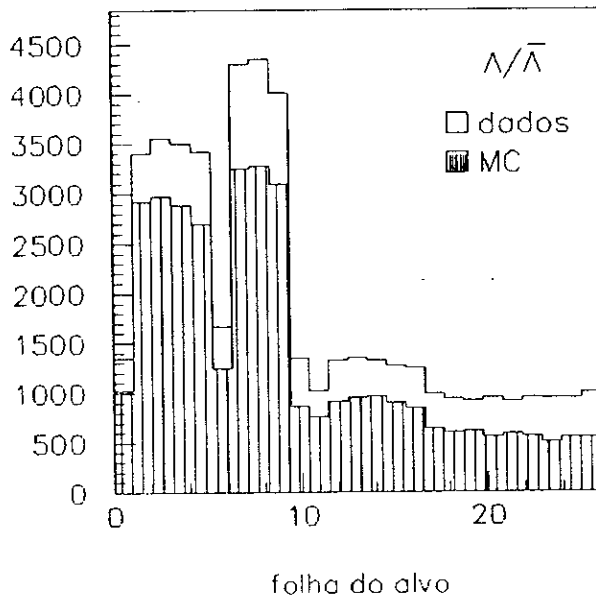
Figura 4.12: Distribuição do Número de \Lambda e \bar{\Lambda} por Folha do Alvo
