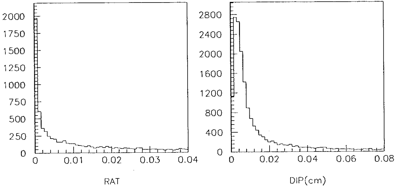
Figura 4.9: Distribuições de RAT e DIP obtidas da Simulação .
