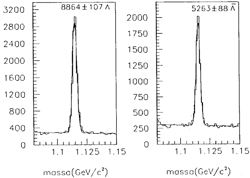
Figura 4.10: Sinais do \Lambda e \bar{\Lambda}
