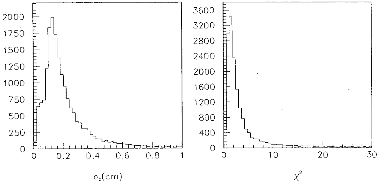
Figura 4.3: Distribuições de \chi^2 e \sigma_z obtidas da Simulação .
