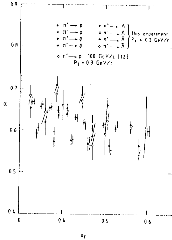
Figura 2.4: \alpha como Função de x_f para p , \bar{p} , \Lambda e \bar{\Lambda} em Interações \pi A a 30 \text{ GeV}/c
